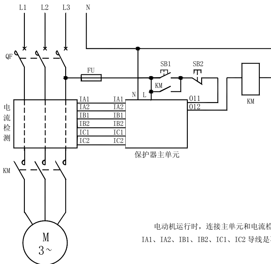
AMDG-□/C0 系列电动机保护器应用电气原理图
