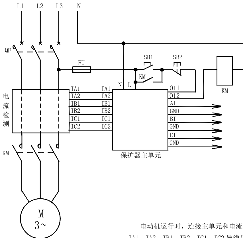
AMDG-□/C1 系列电动机保护器应用电气原理图
