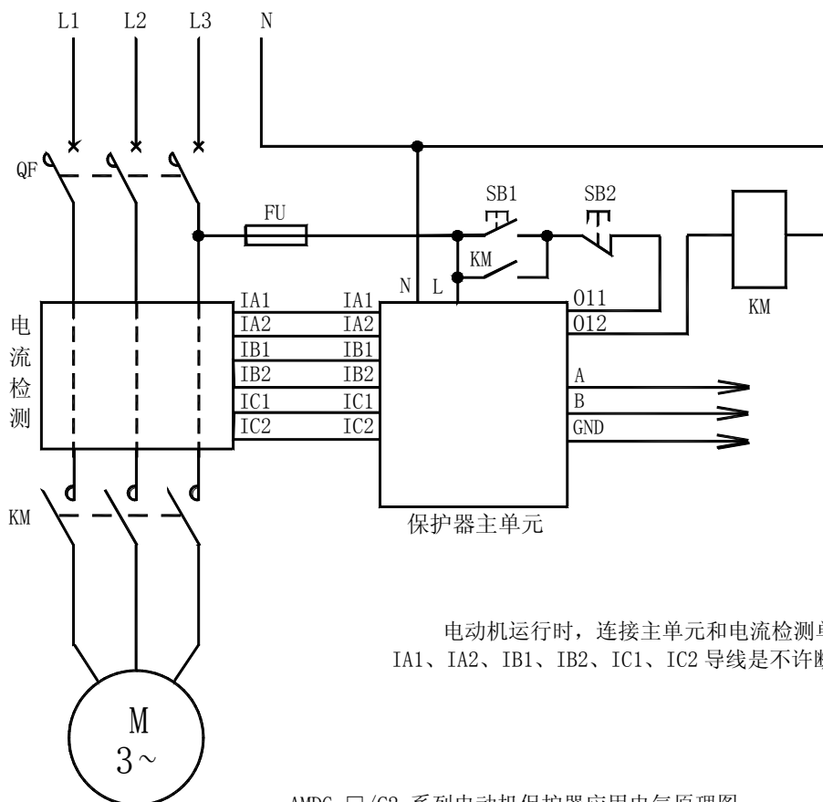
AMDG-□/C2 系列电动机保护器应用电气原理图
