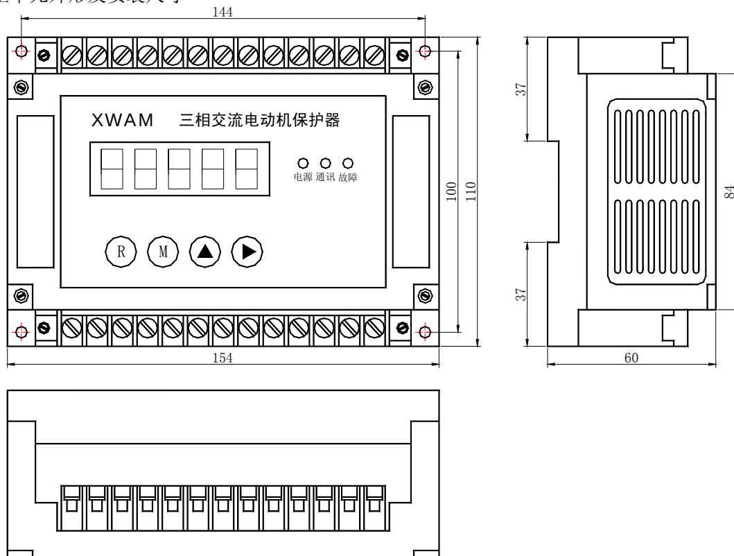
AMDG-□/C2 系列电动机保护器主单元外形及安装孔尺寸
