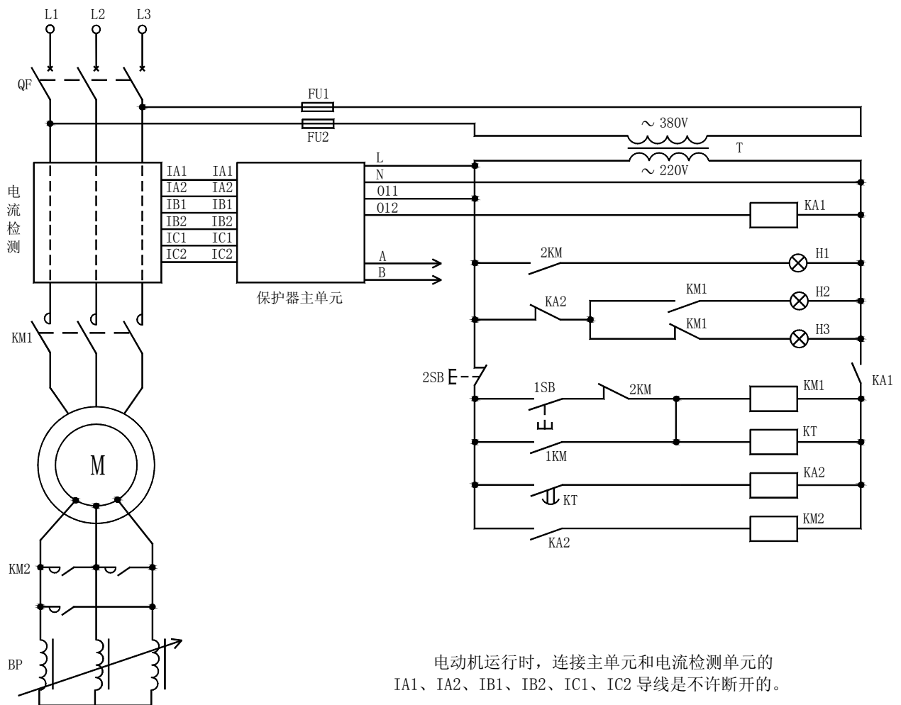
图 1 电动机保护器用于频敏启动控制电气原理图
