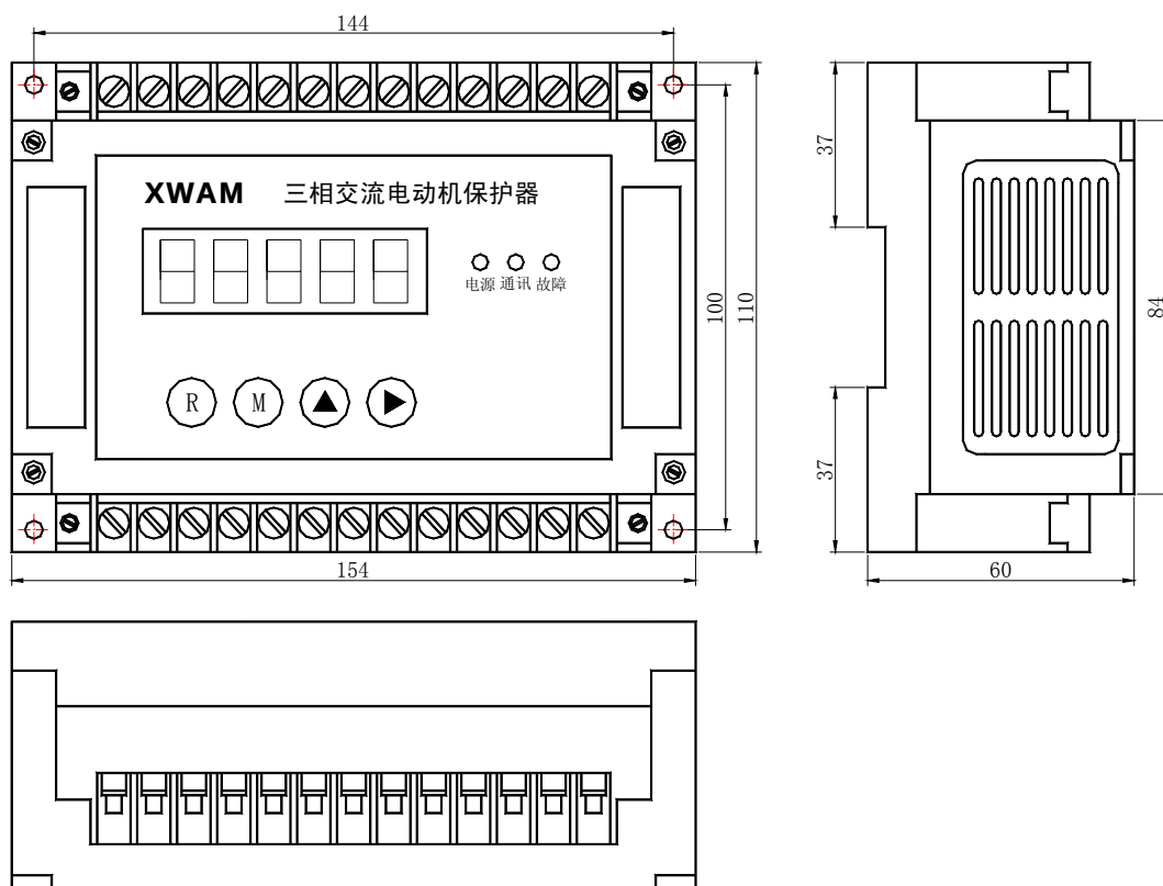
AMDG-□/C4 系列电动机保护器主单元外形及安装孔尺寸
