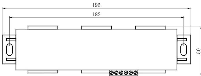
穿线孔直径 \Phi 30\text{mm} 的电流检测单元外形及安装尺寸
