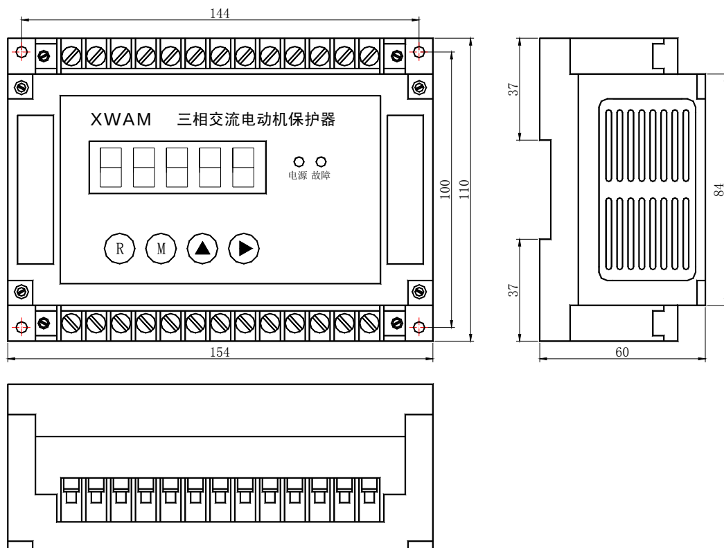
AMDG-□/C5 系列电动机保护器主单元外形及安装孔尺寸
