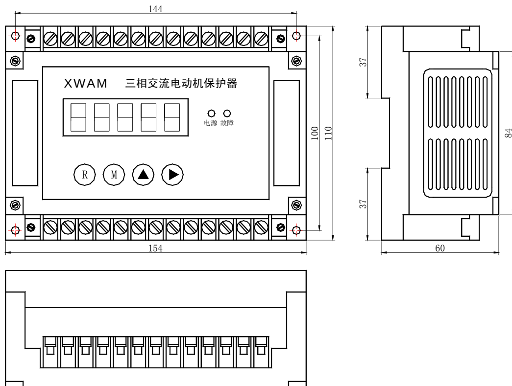
AMDG-□/C7 系列电动机保护器主单元外形及安装孔尺寸
