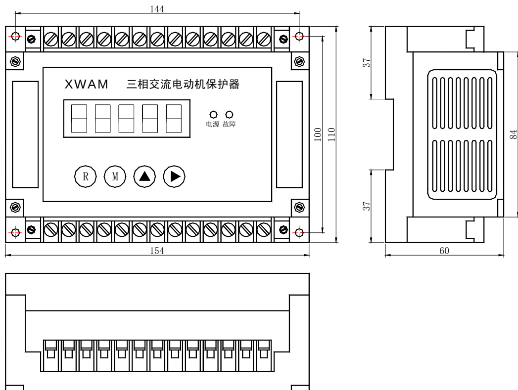
AMDG-□/C8 系列电动机保护器主单元外形及安装孔尺寸
