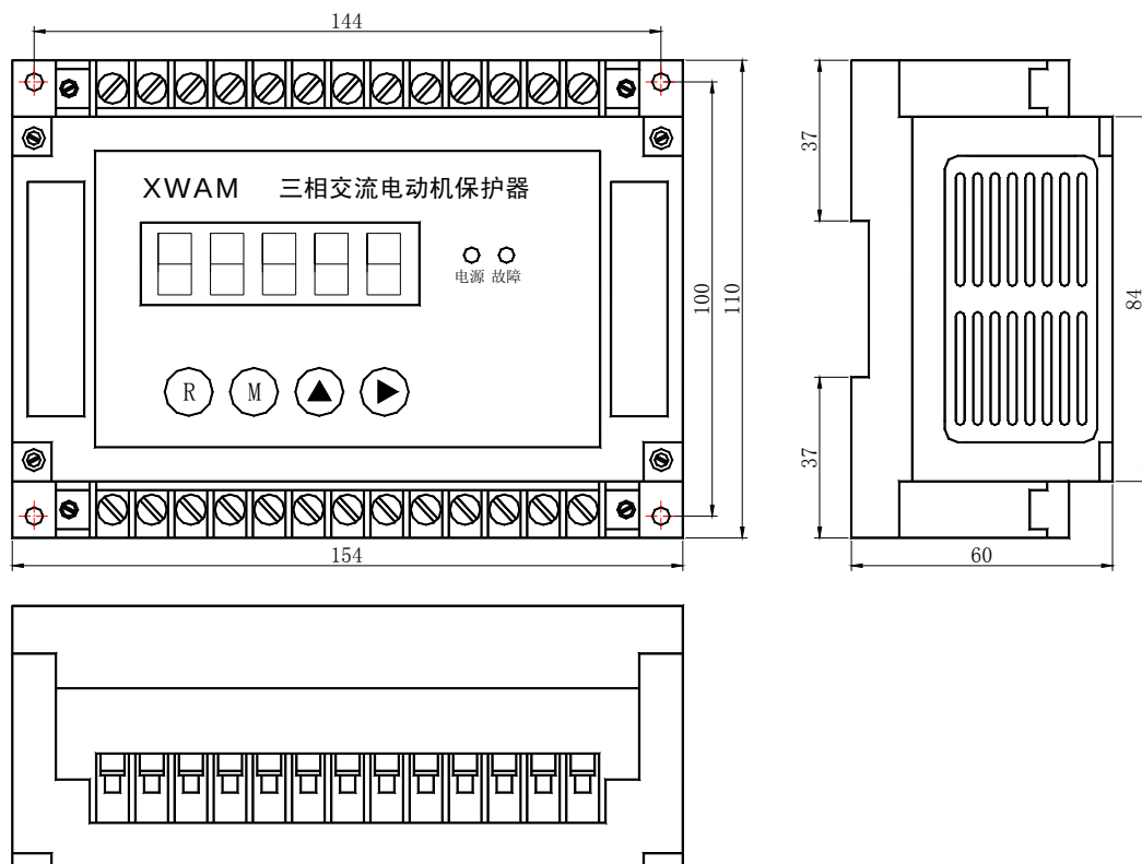
AMDG-□/D7 系列电动机保护器主单元外形及安装孔尺寸
