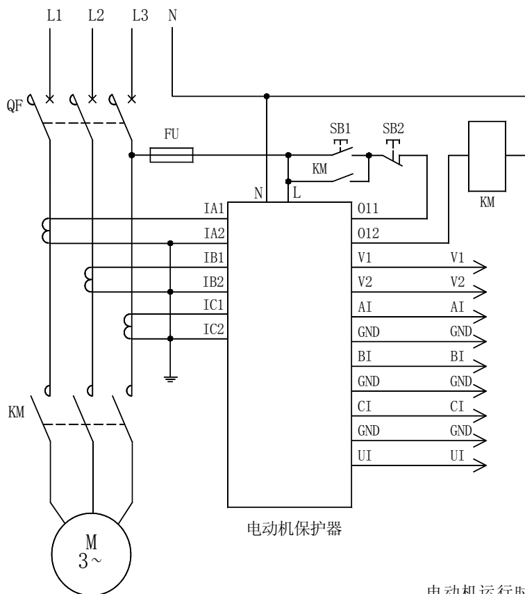
AMDG-X/F1 系列电动机保护器应用电气原理图
