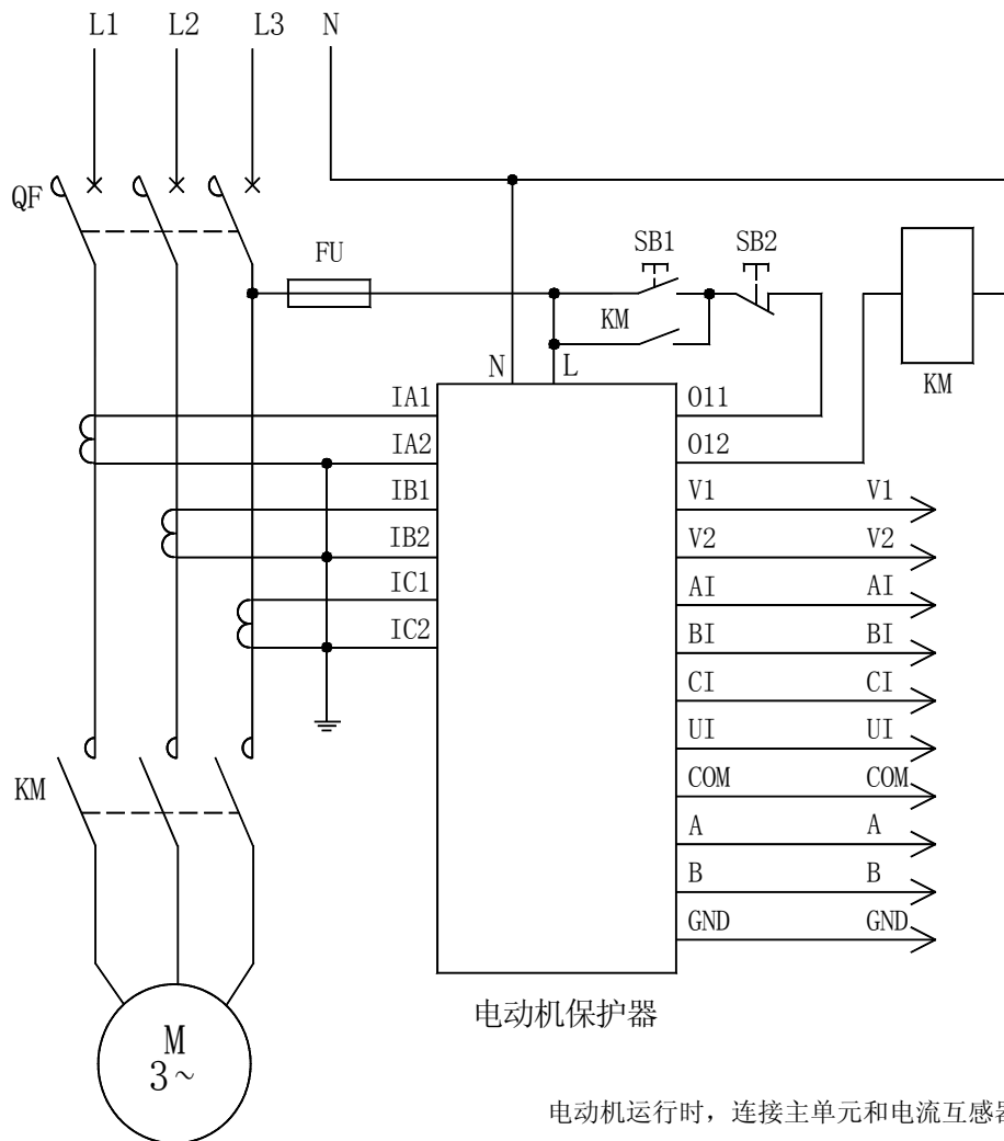
AMDG-X/F4 系列电动机保护器应用电气原理图
