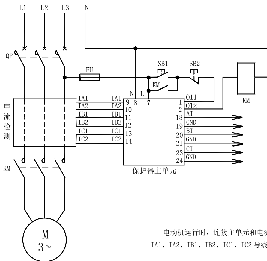
AMDP-□/C1 系列电动机保护器应用电气原理图
