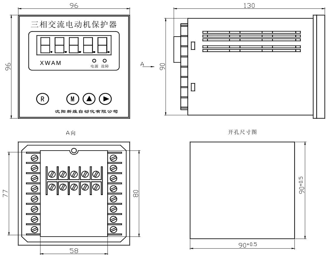
AMDP-□/D0 系列电动机保护器主单元外形及安装孔尺寸
