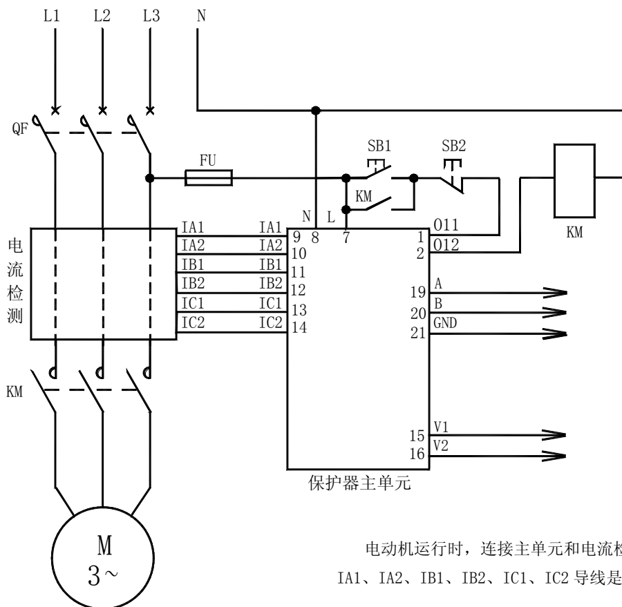
AMDP-□/D2 系列电动机保护器应用电气原理图
