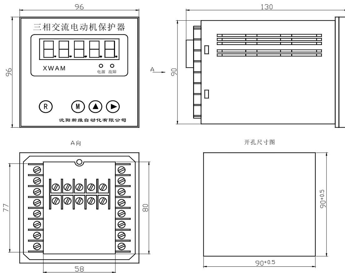
AMDP-X/F4 系列电动机保护器主单元外形及安装孔尺寸
