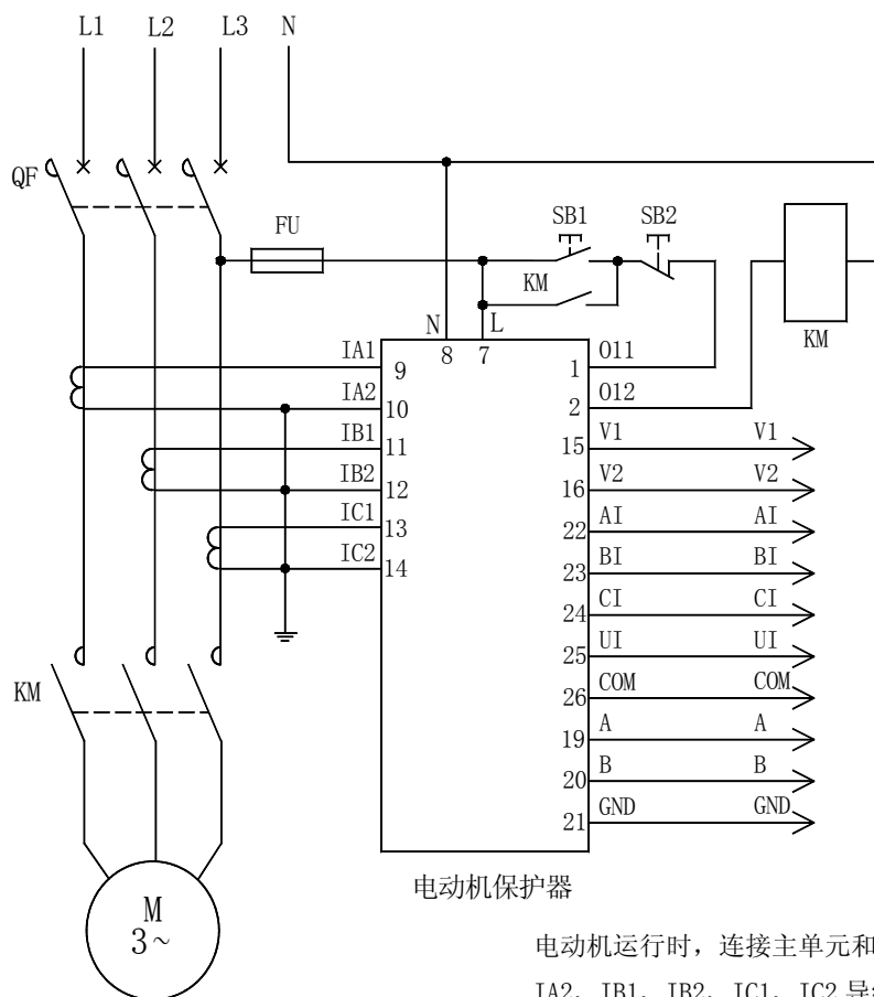
AMDP-X/F4 系列电动机保护器应用电气原理图
