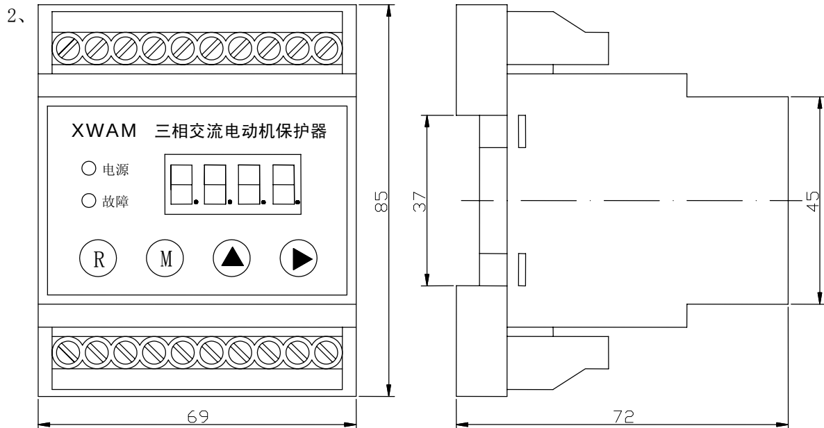
AMDS-□/B 系列电动机保护器主单元外形及安装孔尺寸
