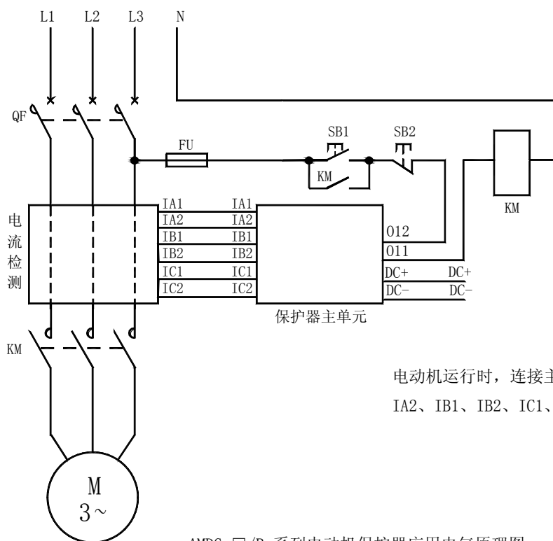
AMDG-□/B 系列电动机保护器应用电气原理图
