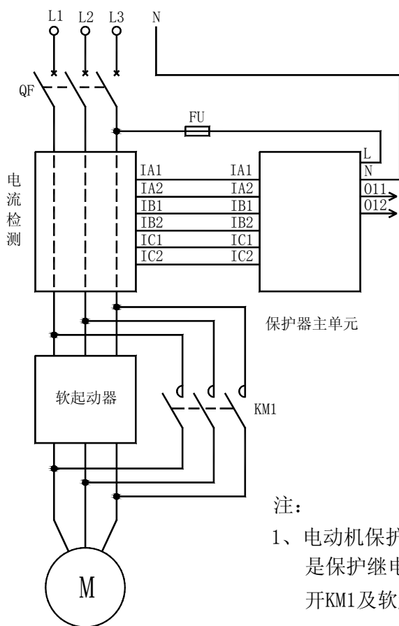
图1 电动机保护器用于软起动控制电气原理图
