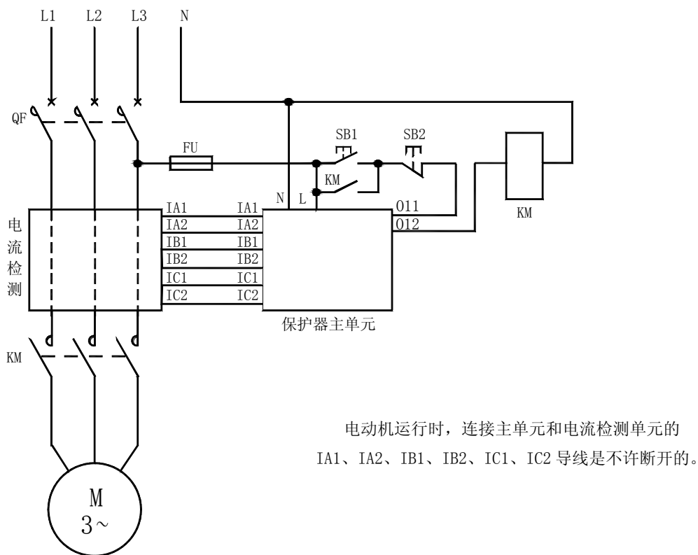
AMDG-□/CO 系列电动机保护器应用电气原理图
