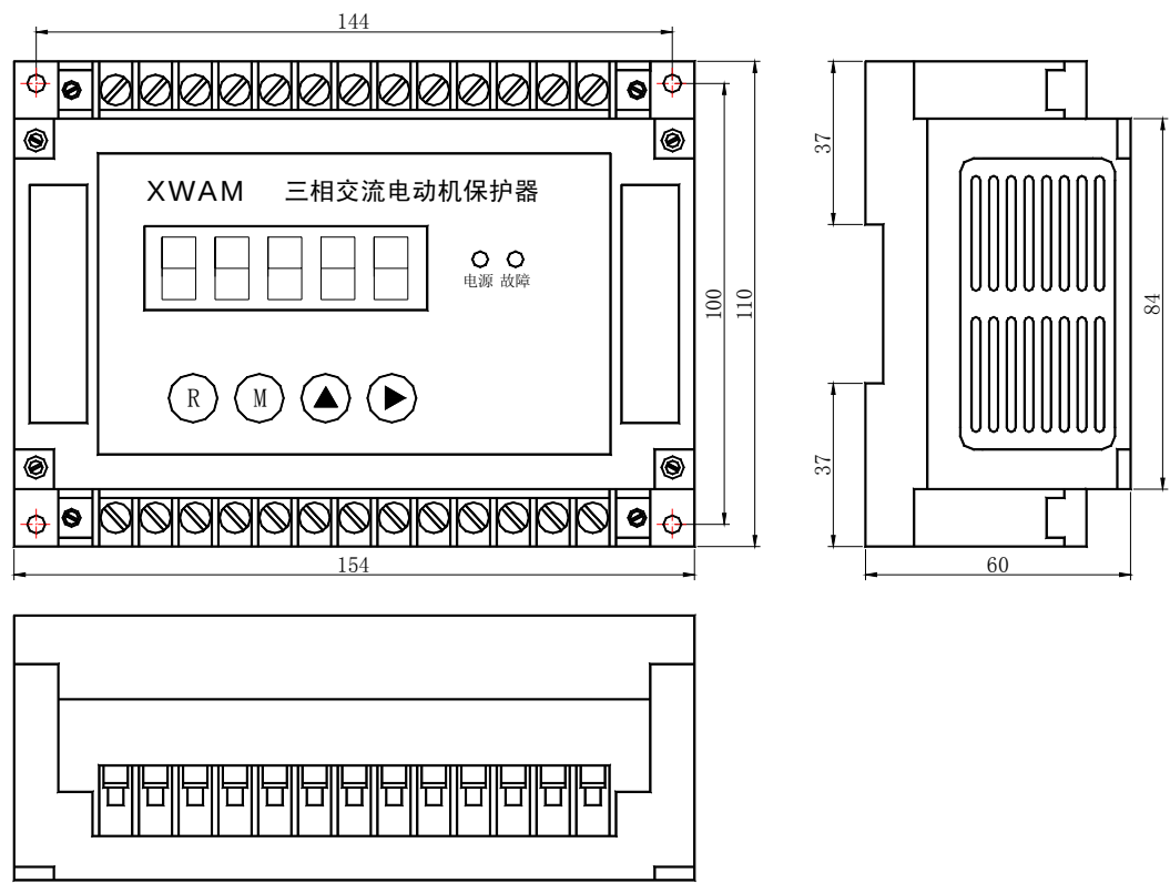
AMDG-□/C1 系列电动机保护器主单元外形及安装孔尺寸
