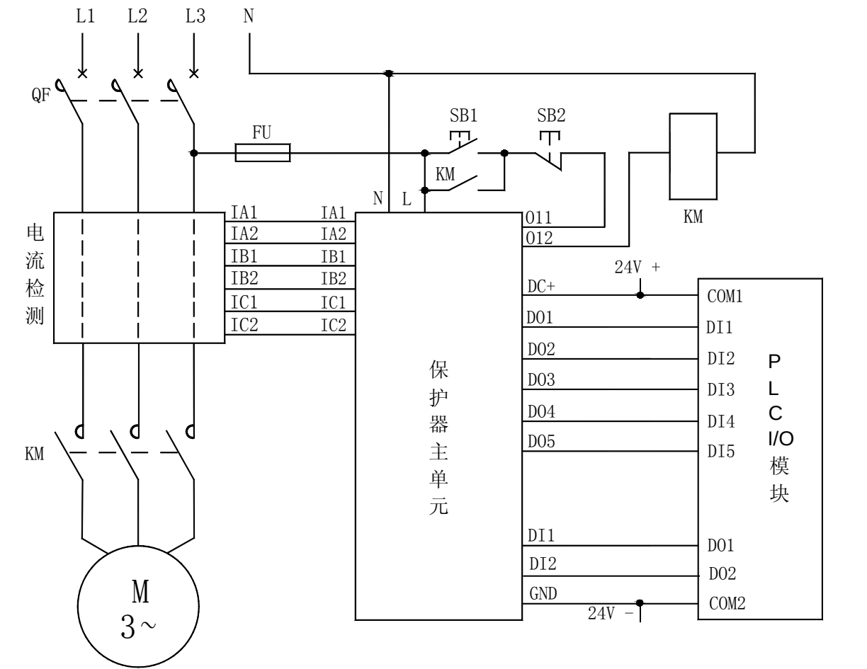
电动机运行时，连接主单元和电流检测单元的 IA1、IA2、IB1、IB2、IC1、IC2 导线是不许断
