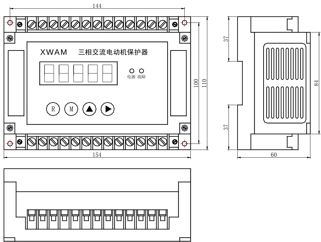
AMDG-□/C6 系列电动机保护器主单元外形及安装孔尺寸
