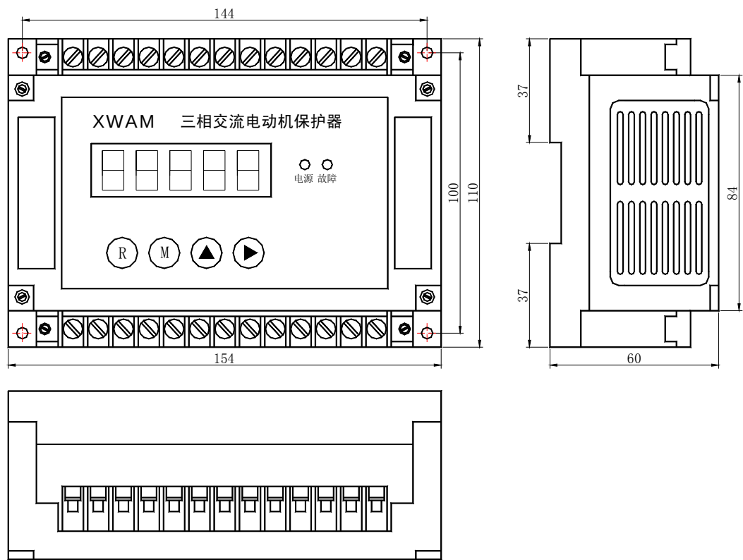
AMDG-□/DO 系列电动机保护器主单元外形及安装孔尺寸
