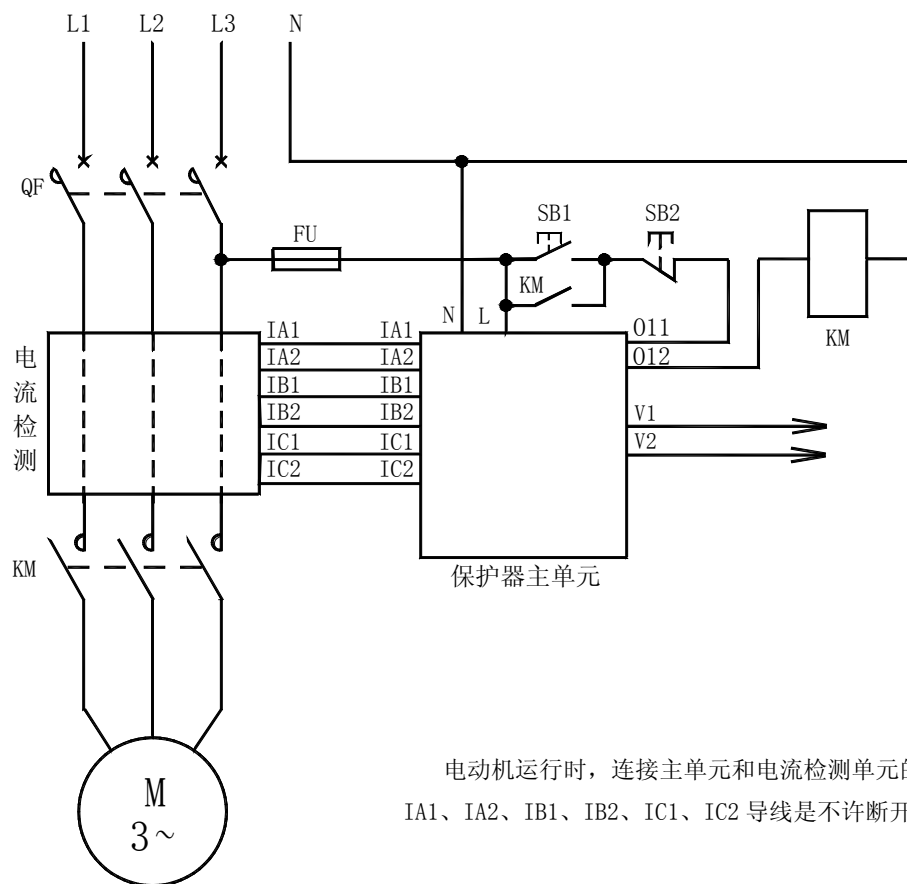
AMDG-□/D0 系列电动机保护器应用电气原理图
