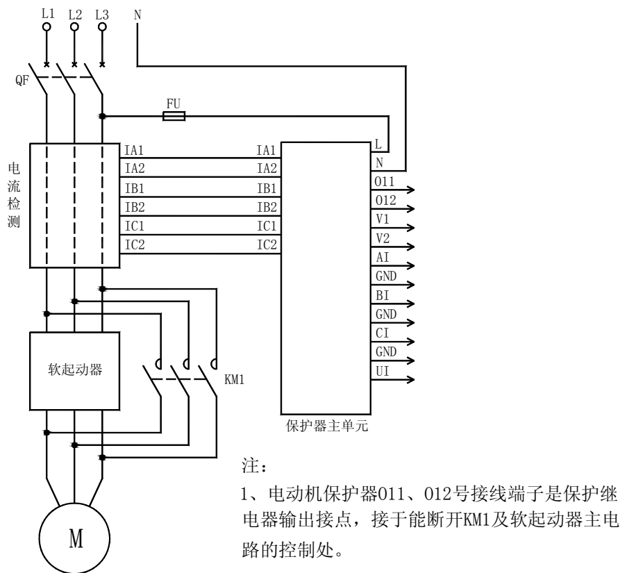
图 1 电动机保护器用于软起动控制电气原理图
