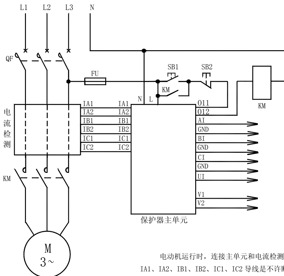
AMDG-□/D1 系列电动机保护器应用电气原理图
