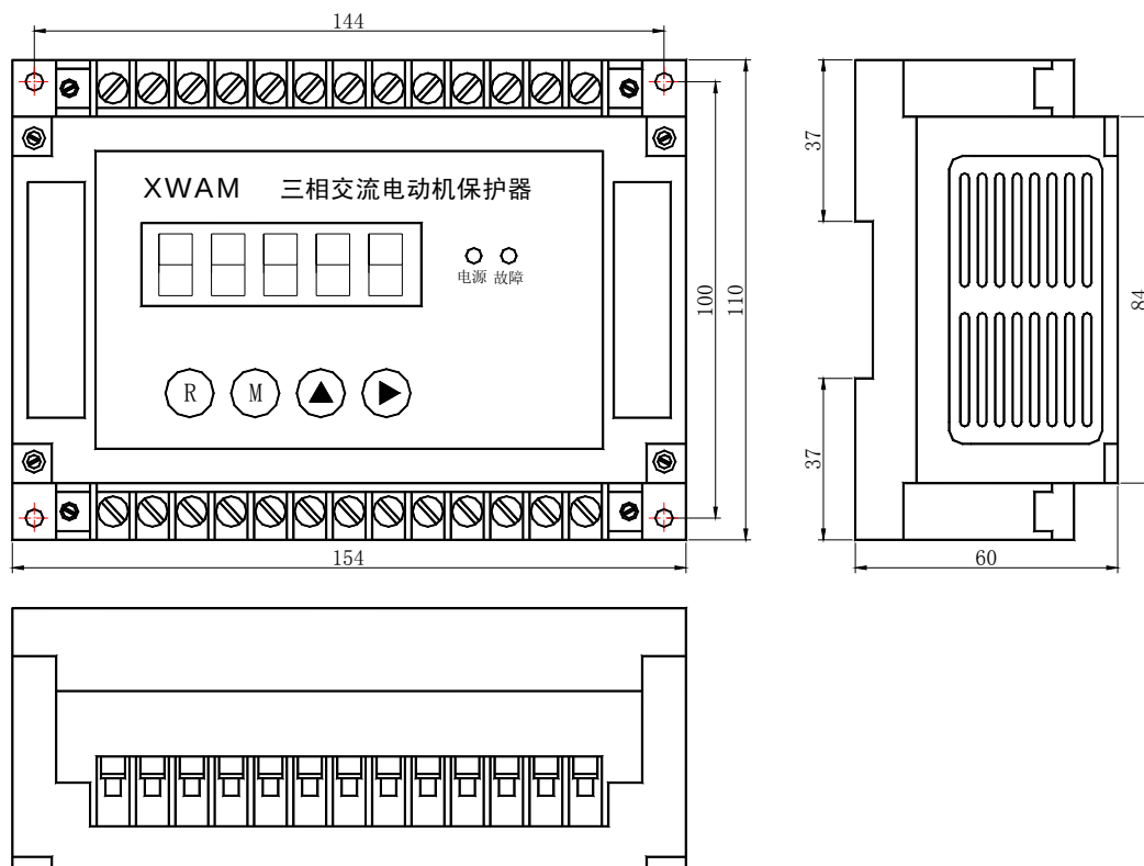
AMDG-□/D1 系列电动机保护器主单元外形及安装孔尺寸
