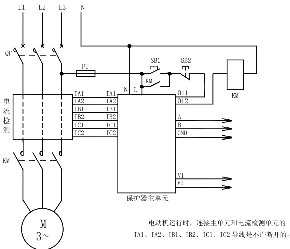
AMDG-□/D3 系列电动机保护器应用电气原理图
