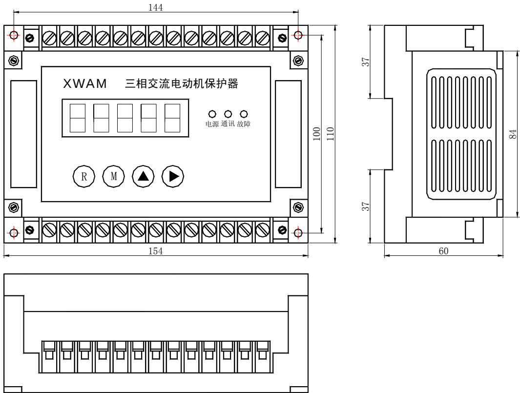
AMDG-□/D4 系列电动机保护器主单元外形及安装孔尺寸
