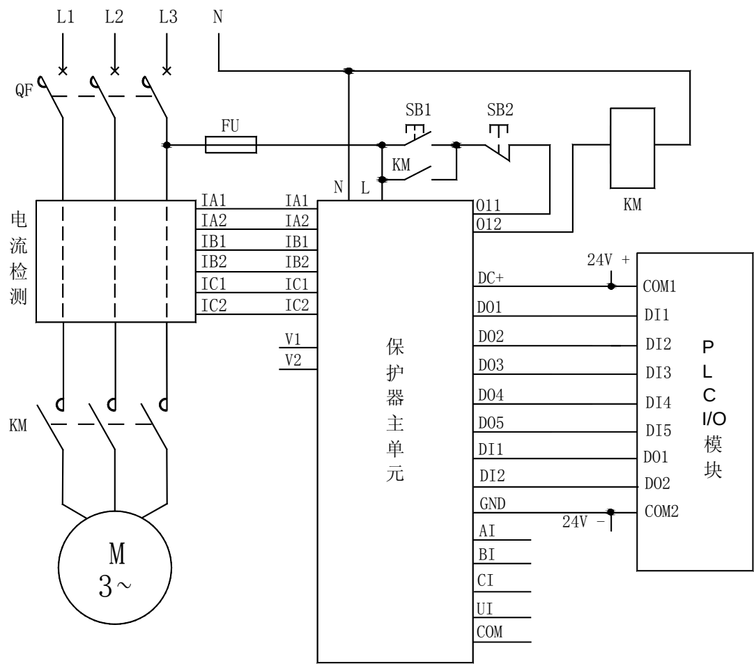
电动机运行时，连接主单元和电流检测单元的 IA1、IA2、IB1、IB2、IC1、IC2 导线是不许断
