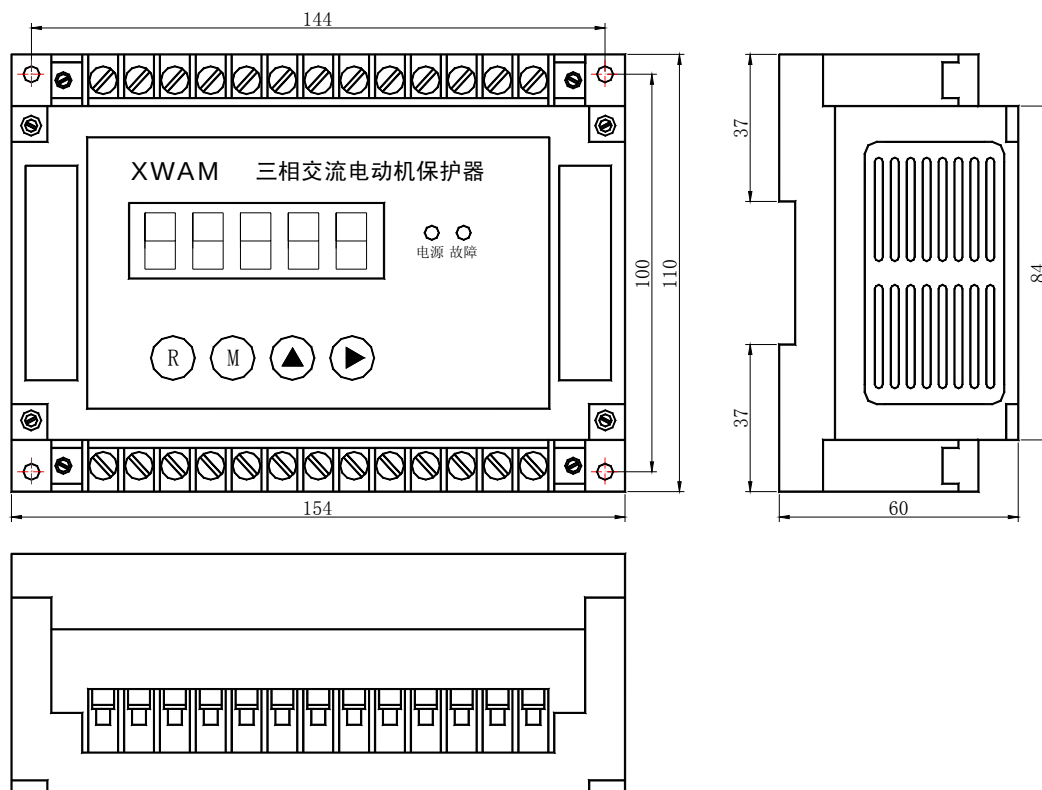
AMDG-X/E0 系列电动机保护器主单元外形及安装孔尺寸
