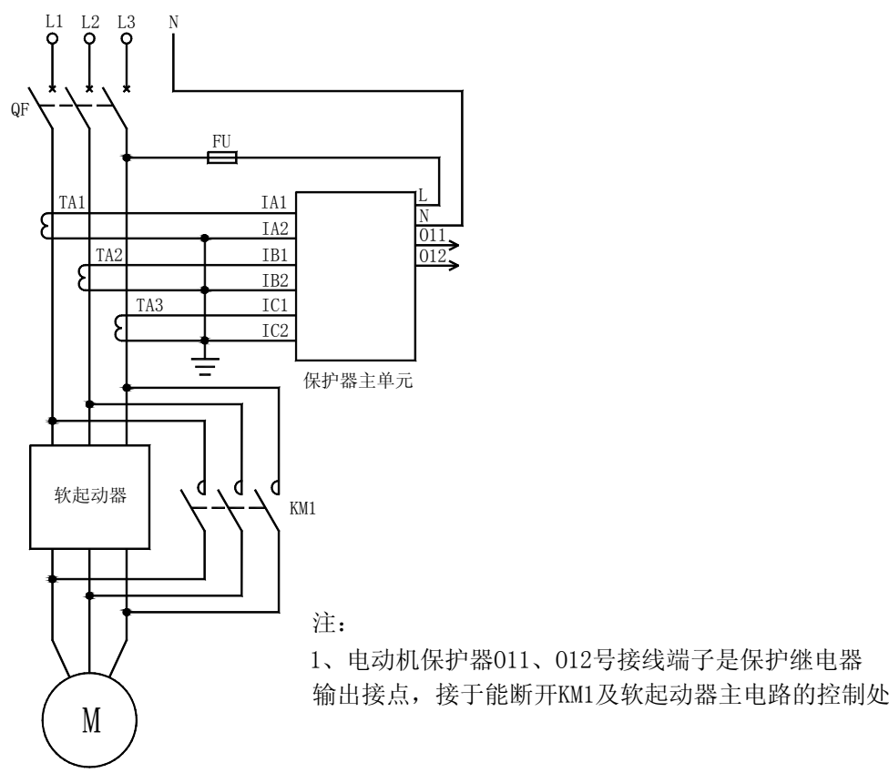
图 1 电动机保护器用于软起动控制电气原理图
