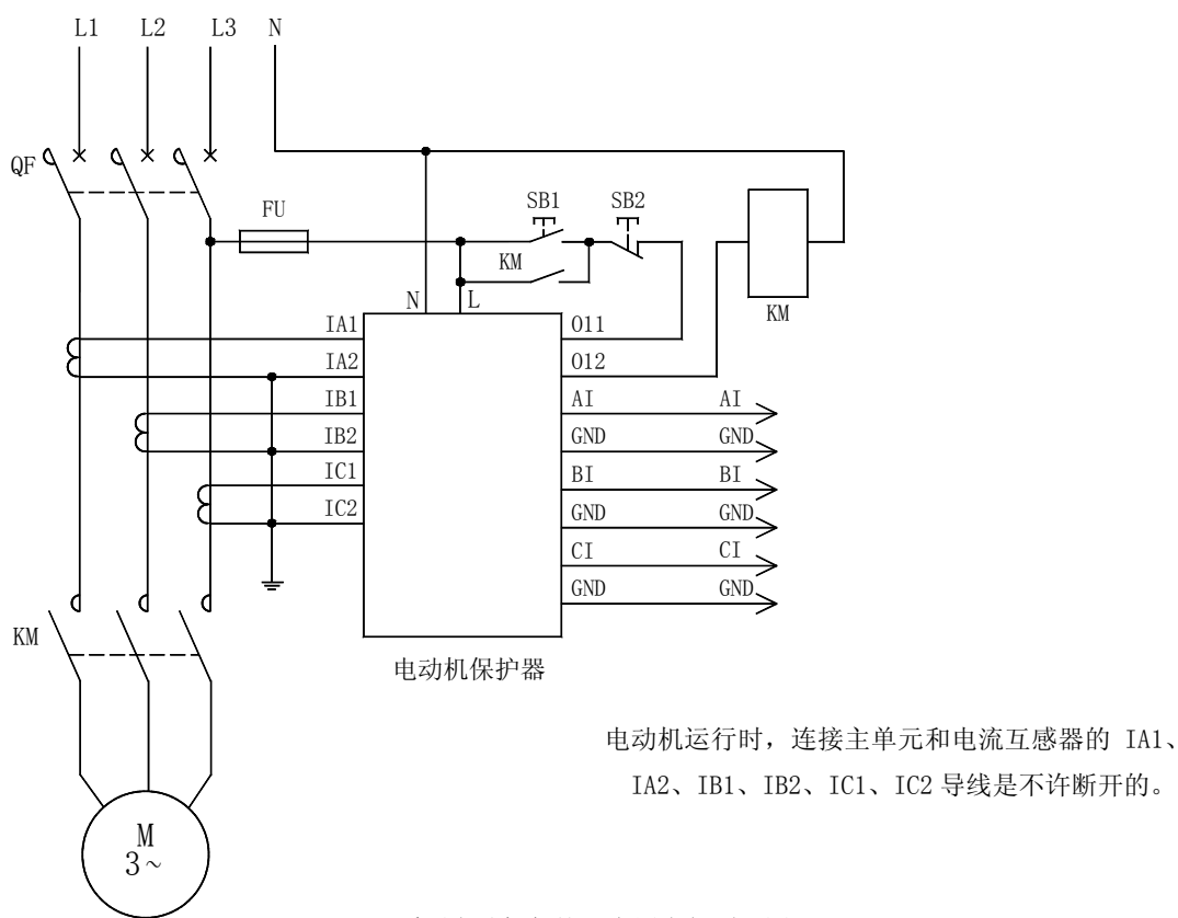
AMDG-X/E1 系列电动机保护器应用电气原理图
