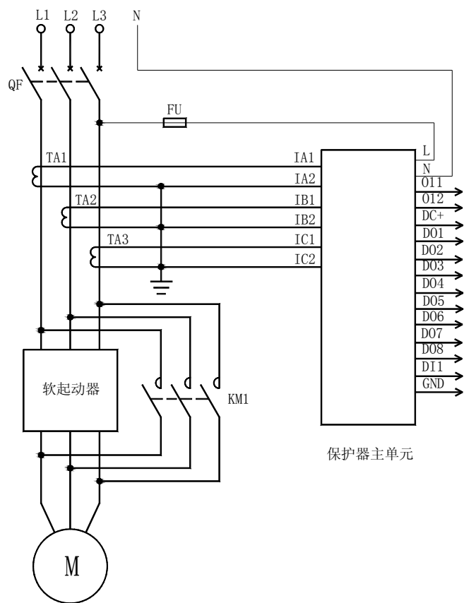
图 1 电动机保护器用于软启动控制电气原理图
