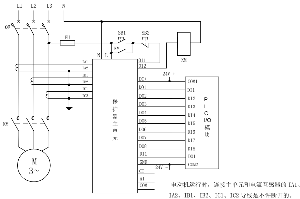
AMDG-X/E7 系列电动机保护器应用电气原理图
