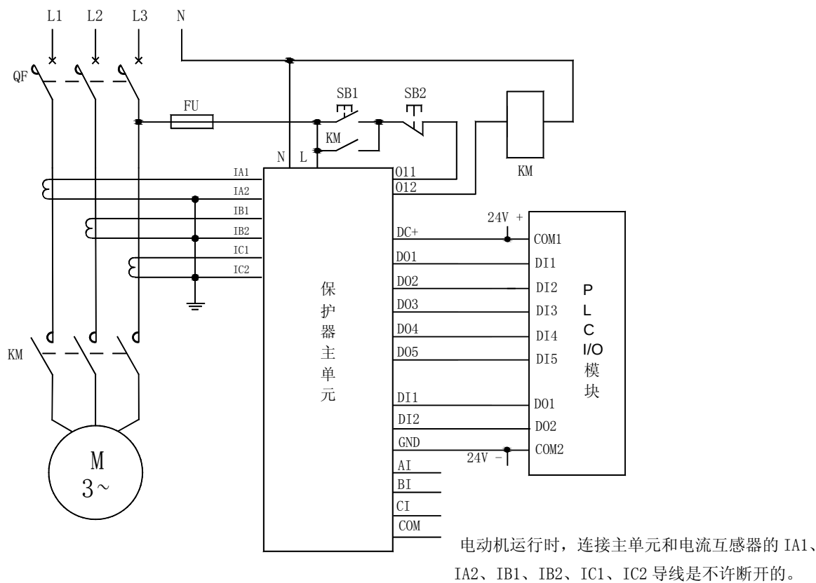
AMDG-X/E8 系列电动机保护器应用电气原理图
