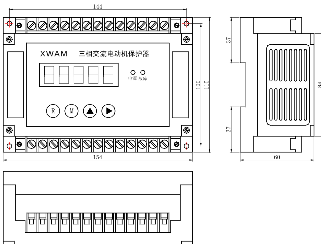
AMDG-X/F0 系列电动机保护器主单元外形及安装孔尺寸
