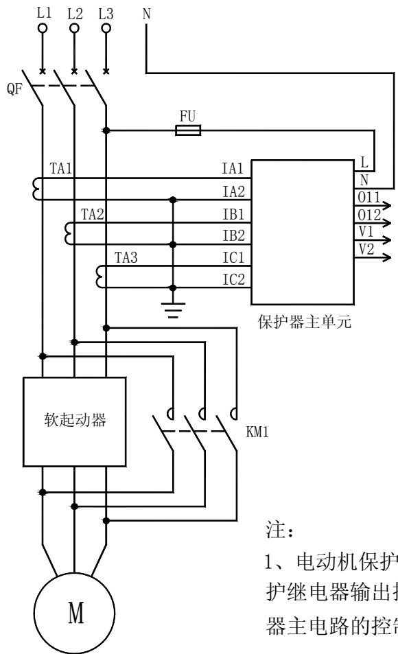
图 1 电动机保护器用于软起动控制电气原理图
