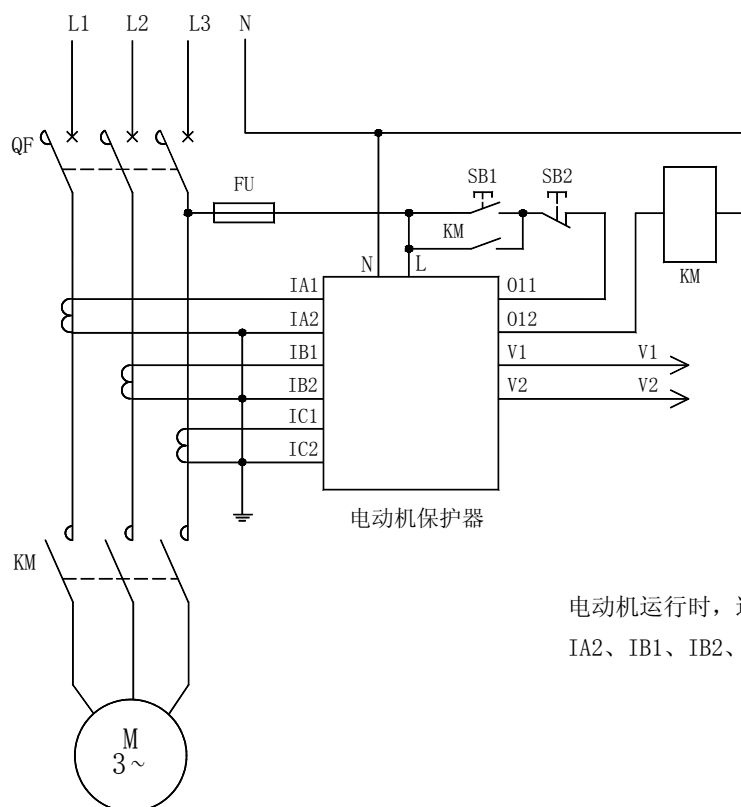
AMDG-X/F0 系列电动机保护器应用电气原理图
