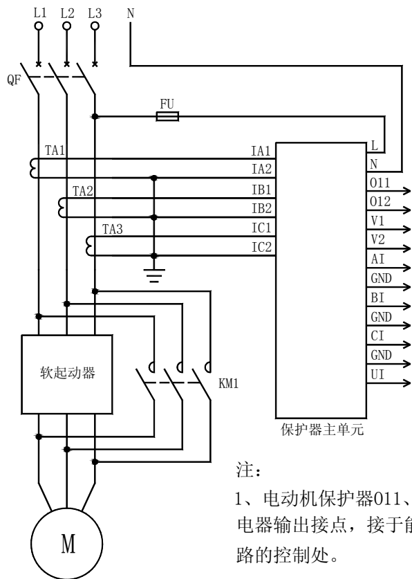
图 1 电动机保护器用于软起动控制电气原理图
