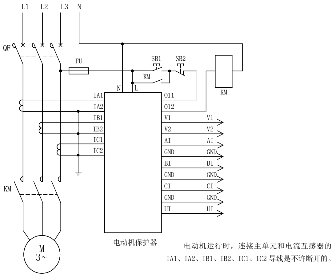
AMDG-X/F1 系列电动机保护器应用电气原理图
