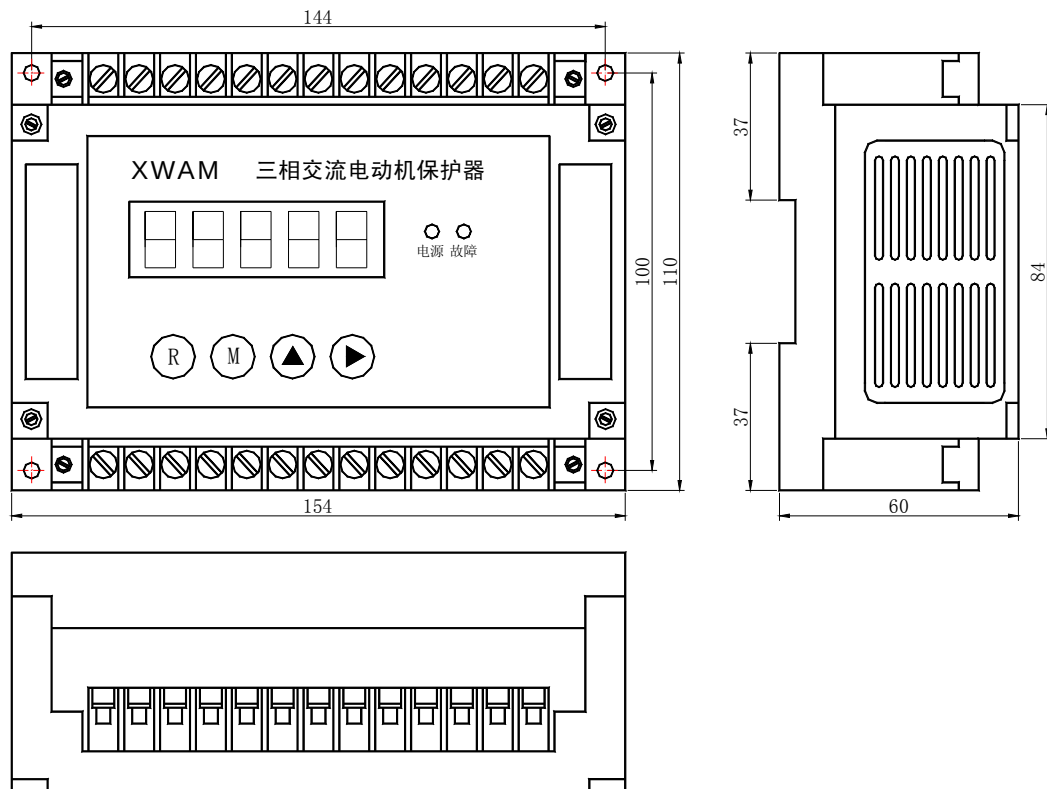
AMDG-X/F1 系列电动机保护器主单元外形及安装孔尺寸
