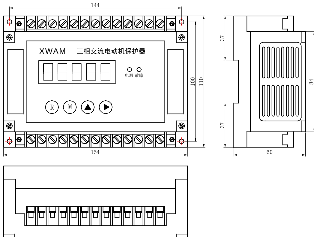
AMDG-X/F5 系列电动机保护器主单元外形及安装孔尺寸
