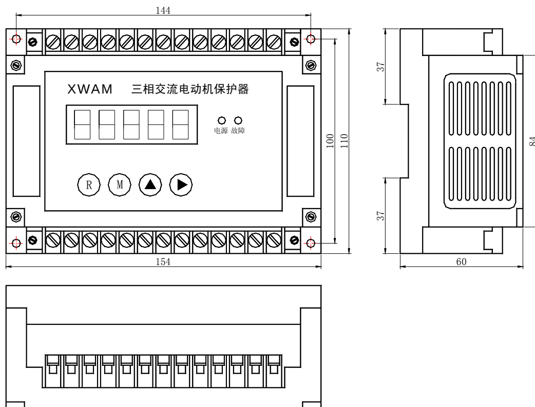
AMDG-X/F6 系列电动机保护器主单元外形及安装孔尺寸
