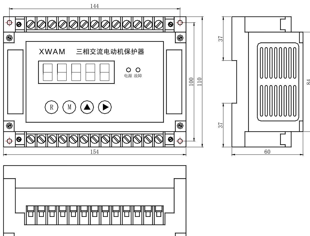
AMDG-X/F8 系列电动机保护器主单元外形及安装孔尺寸
