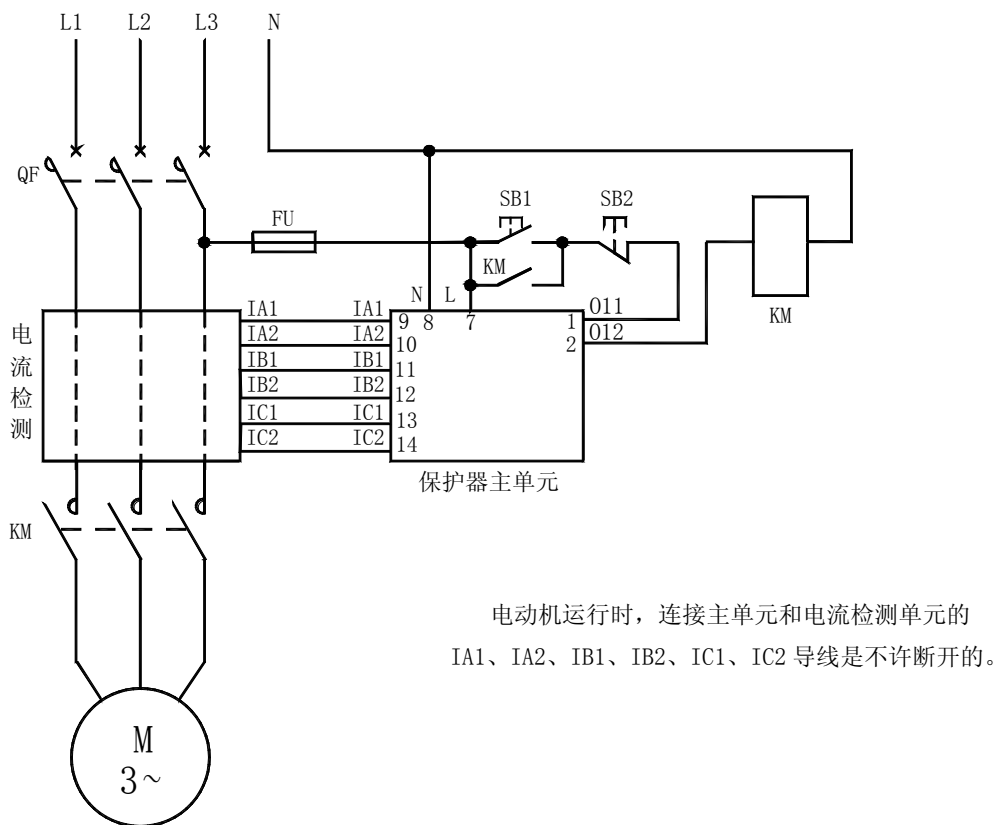
AMDP-□/C0 系列电动机保护器应用电气原理图
