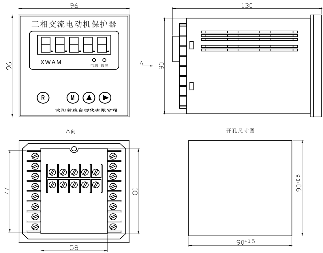
AMDP-□/C1 系列电动机保护器主单元外形及安装孔尺寸
