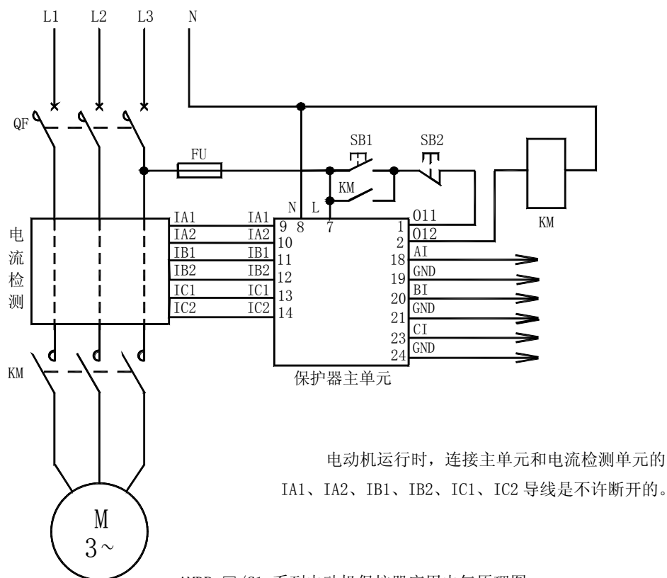
AMDP-□/C1 系列电动机保护器应用电气原理图
