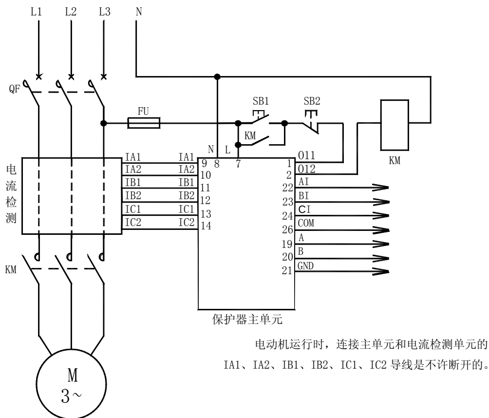
AMDP-□/C4 系列电动机保护器应用电气原理图
