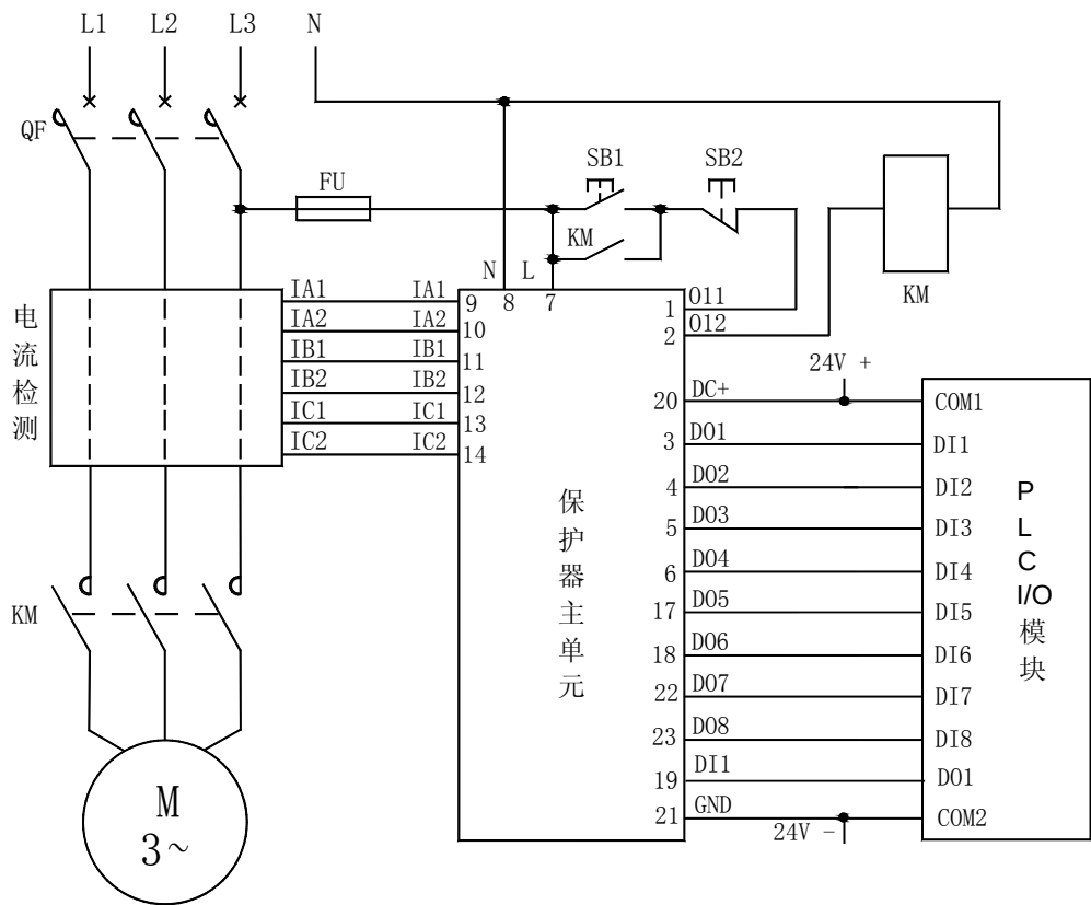
电动机运行时，连接主单元和电流检测单元的 IA1、IA2、IB1、IB2、IC1、IC2 导线是不许断
