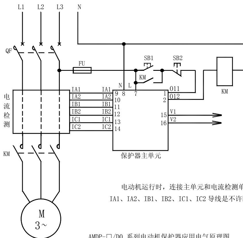
AMDP-□/D0 系列电动机保护器应用电气原理图
