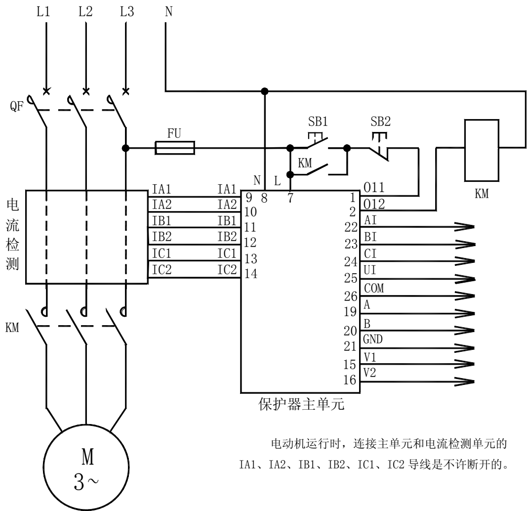
AMDP-□/D4 系列电动机保护器应用电气原理图
