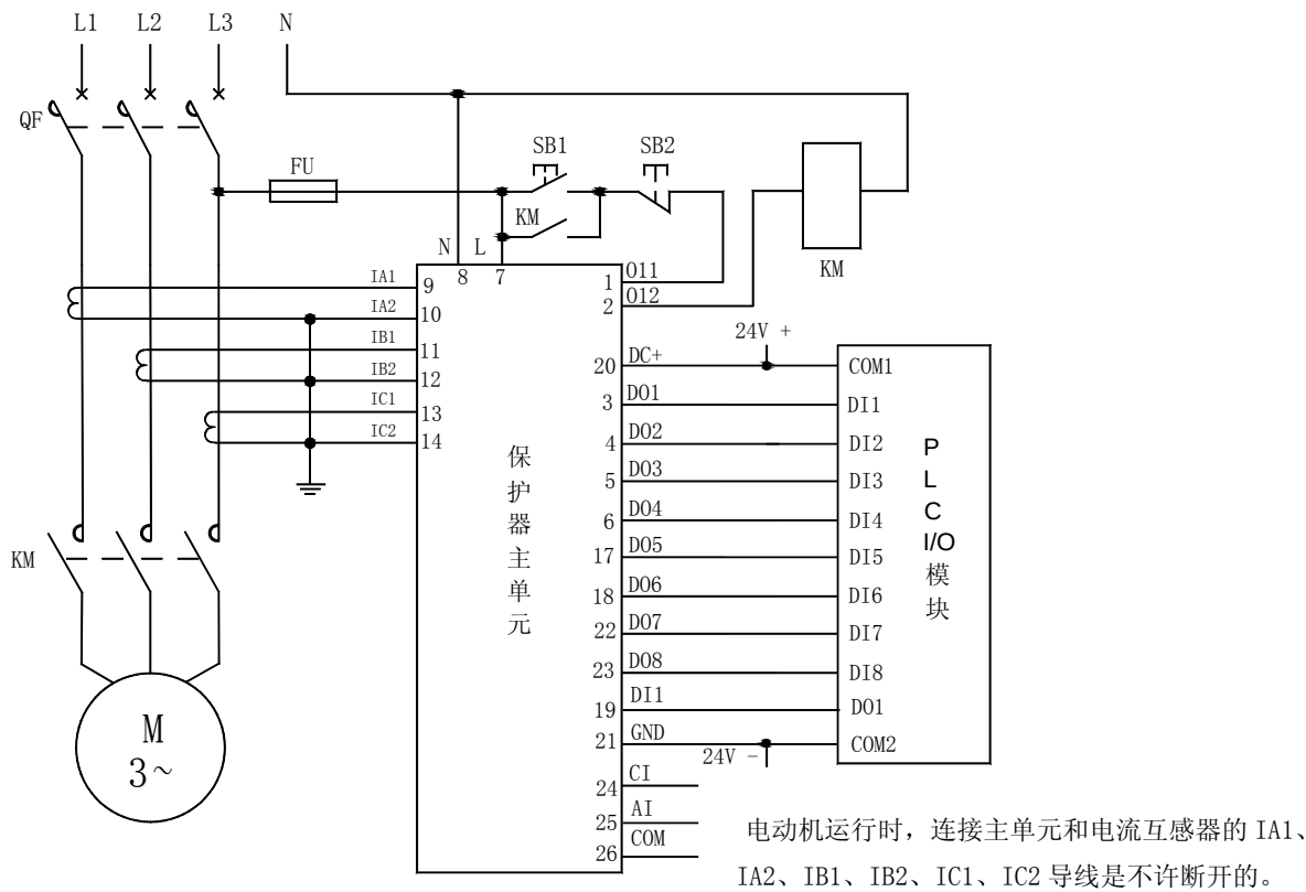
AMDP-X/E7 系列电动机保护器应用电气原理图
