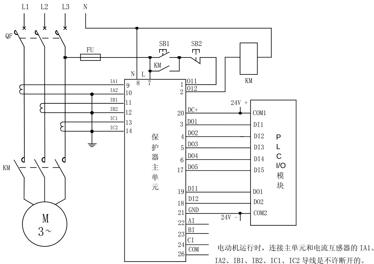
AMDP-X/E8 系列电动机保护器应用电气原理图
