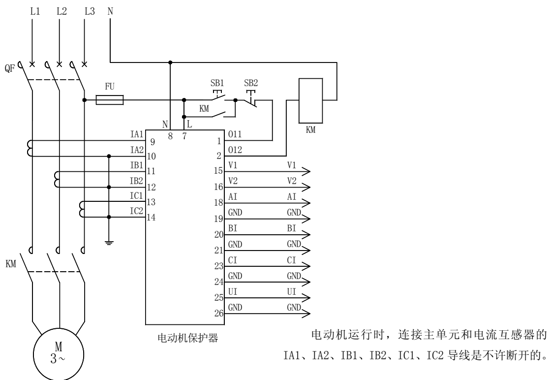
AMDP-X/F1 系列电动机保护器应用电气原理图
