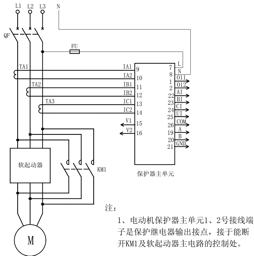
图 1 电动机保护器用于软起动控制电气原理图
