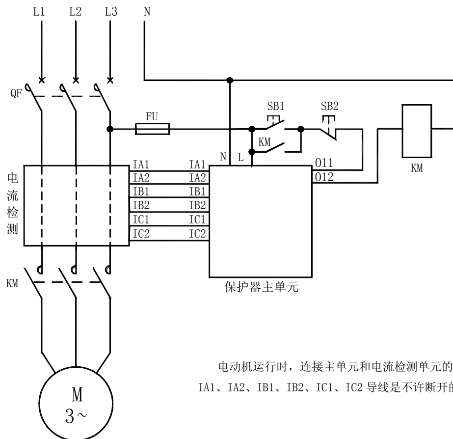
AMDS-□/D 系列电动机保护器应用电气原理图
