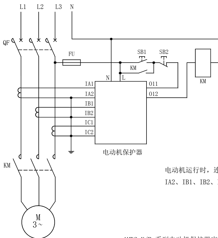
AMDS-X/F 系列电动机保护器应用电气原理图
