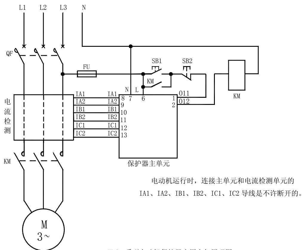
AMDT-□/C 系列电动机保护器应用电气原理图
