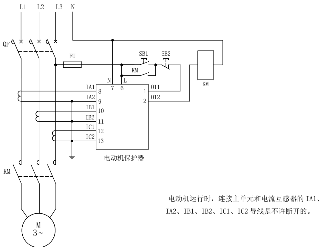
AMDT-X/E 系列电动机保护器应用电气原理图
