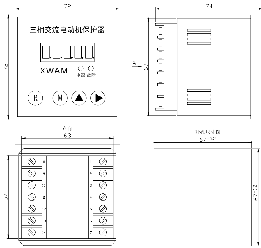
AMDT-X/E 系列电动机保护器主单元外形及安装孔尺寸
