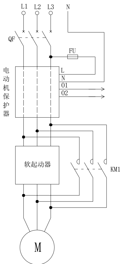
图 1 电动机保护器用于软起动控制电气原理图
