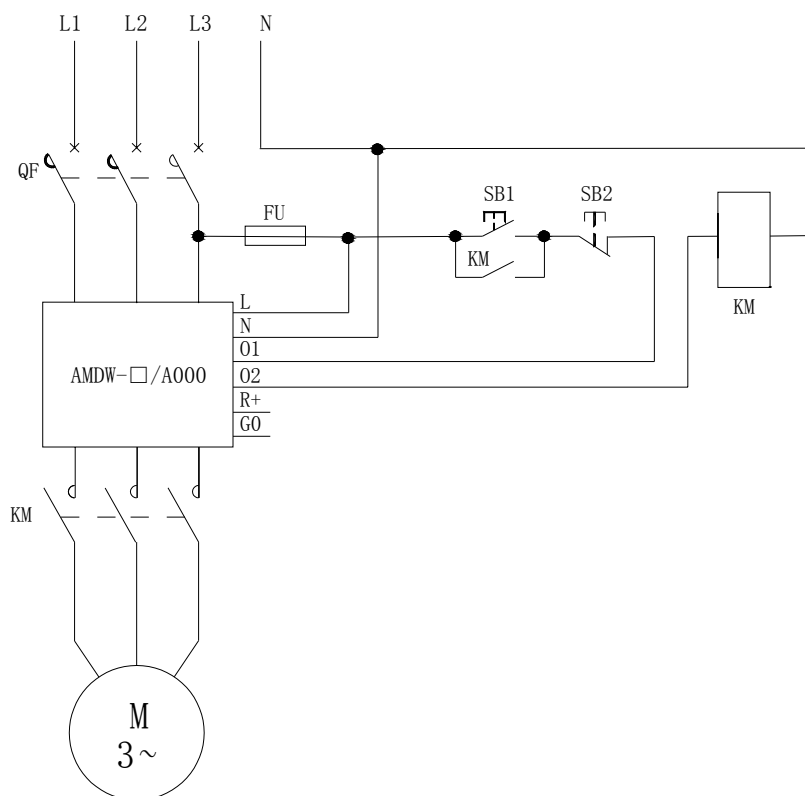
AMDW-□/B 系列电动机保护器应用电气原理图
